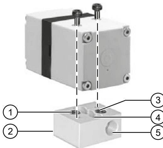
Abb. 4: Proportional-Druckregelventil, auf Einzelanschlussplatte oder Batterieleiste montierbar
