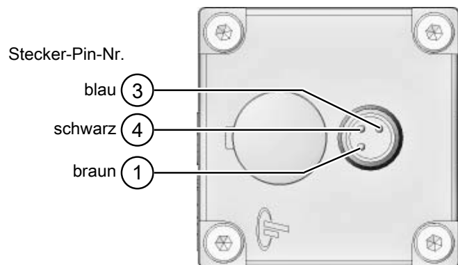
Abb. 5: Anschlussschema
